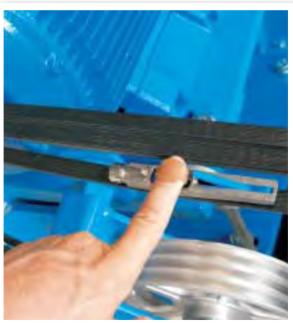
Téster Optikrik de Optibelt
