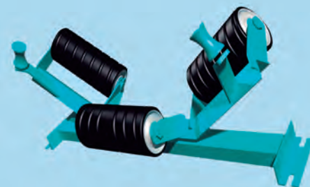
AUTOCENTRANTE DESPLAZADO
